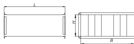
Пластинчатый шумоглушитель с обтекателем
